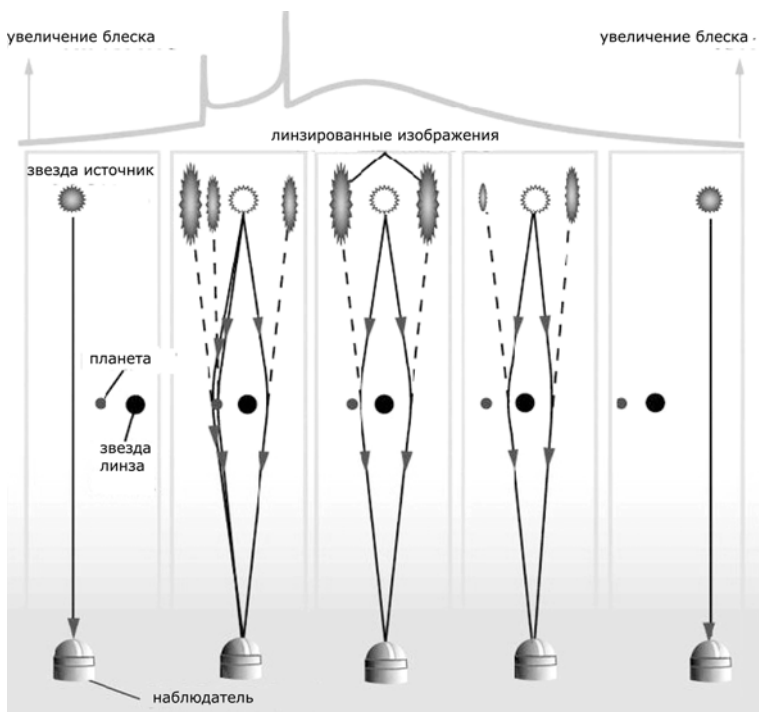
Рис. 8.1. Эффект микролинзирования на двойной линзе. Наличие спутника (планеты) приводит к появлению на кривой блеска дополнительных пиков яркости (кривая вверх).
