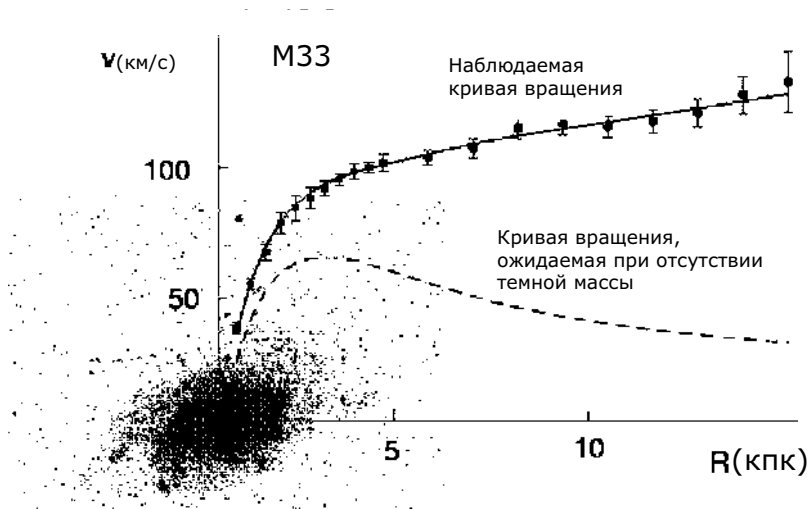
Рис. 11.8. Влияние темного массивного гало на кривую вращения галактик (на примере M33).
