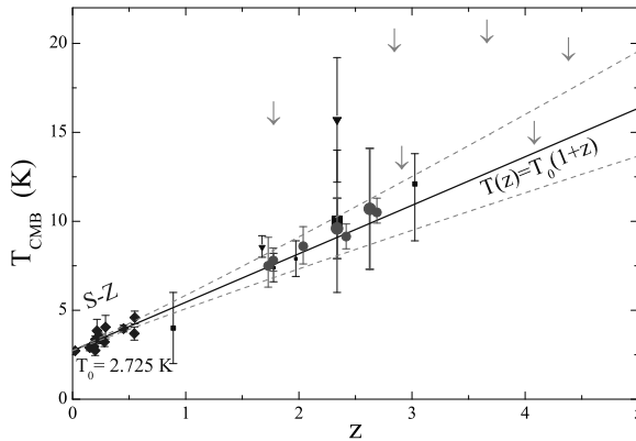
Рис. 12.10. Зависимость температуры реликтового излучения от красного смещения. Определение T_{cmb} на малых z проводится по эффекту Сюняева-Зельдовича на скоплениях галактик, а на больших z — по измерениям линий поглощения атомов \text{C I} и молекул \text{CO} в спектрах далеких квазаров. Сплошная прямая показывает теоретическую зависимость T(z) = T_0(1+z) , пунктир — допустимые ошибки фитирования данных методом наименьших квадратов. Рис. из работы Иванчик А.В. и др. 2011 .
