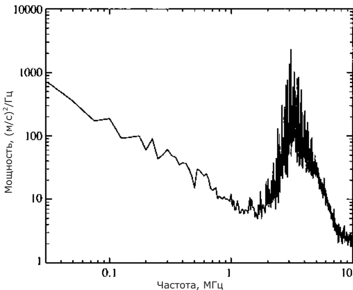
Рис. 5.10. Пример спектра мощности низкого разрешения [(\text{м/с})^2/\text{Гц}] солнечных колебаний 1996 г. в эксперименте GOLF со спутника SOHO. Частоты линий между 2 и 7 МГц соответствуют различным p -модам 5-минутных колебаний Солнца.
