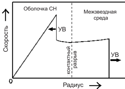
Рис. 9.7. Формирование ударных волн к центру звезды и от звезды при сверхзвуковом расширении остатка сверхновой в межзвездной среде.
