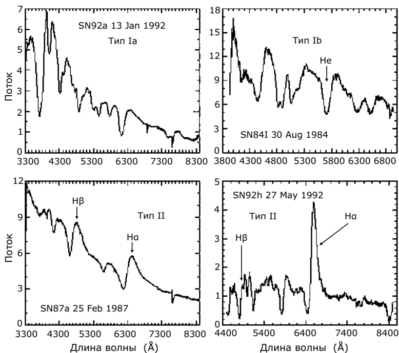
Рис. 9.3. Спектры сверхновых различных типов. В спектрах (особенно у SN II) хорошо видны профили линий типа P Cyg (эмиссия в красном крыле и абсорбция в голубом крыле линии), свидетельствующие о мощной расширяющейся оболочке, как у самых горячих звезд. Ширина линий соответствует скорости расширения 10–30 тыс. км/с.
